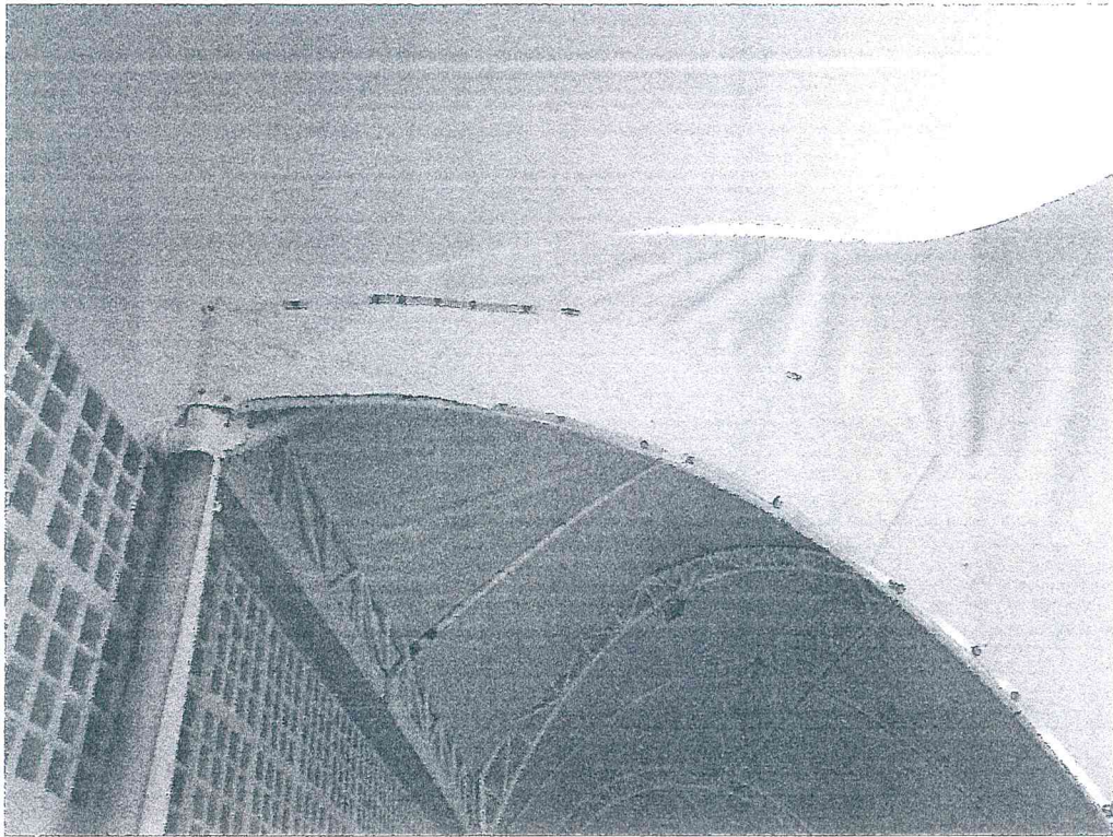
Foto 04: Oxidação das soldas ( Realizar reparos)
