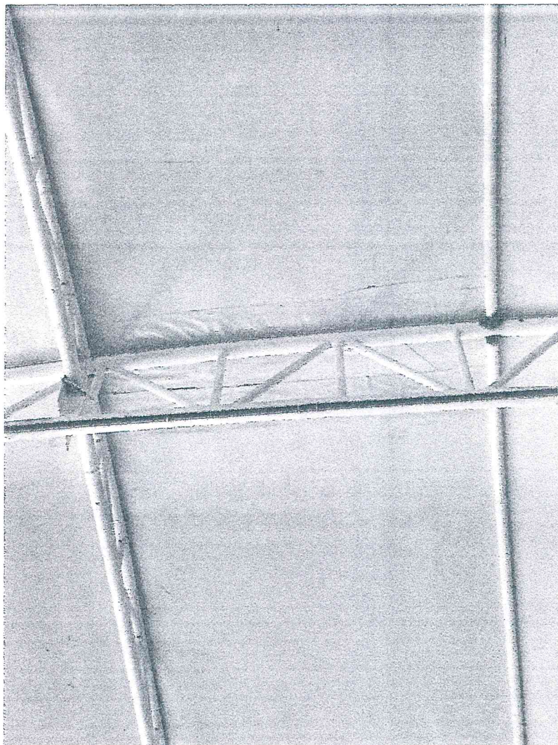
Foto 05: Oxidação das soldas (Realizar reparos) e emendas na lona
